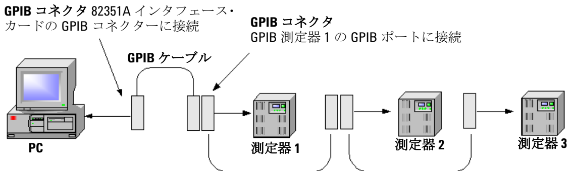
例: 複数の測定器の接続
